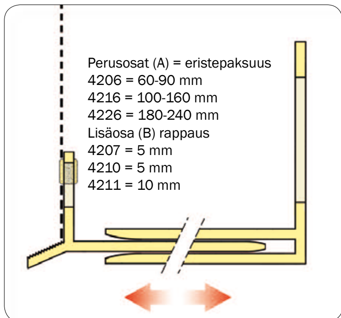
Alumiini / rst profiilit
